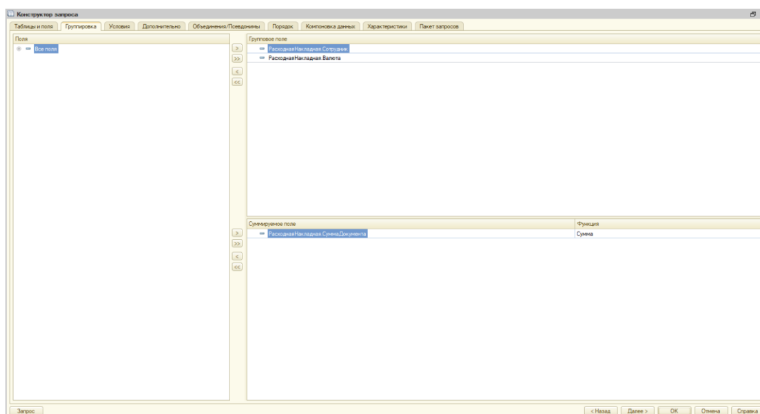
Рисунок 27 – Вкладка «Группировка»
