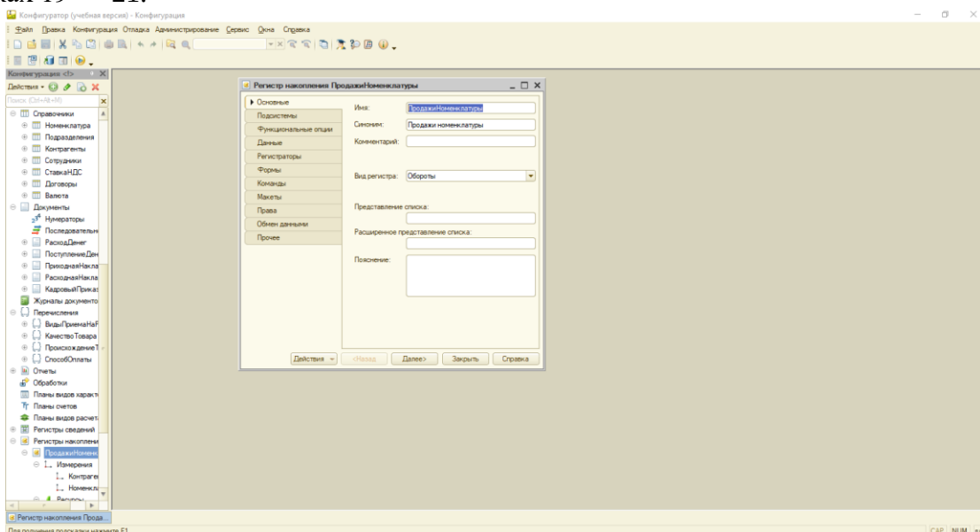
Рисунок 19 – Регистр накоплений
