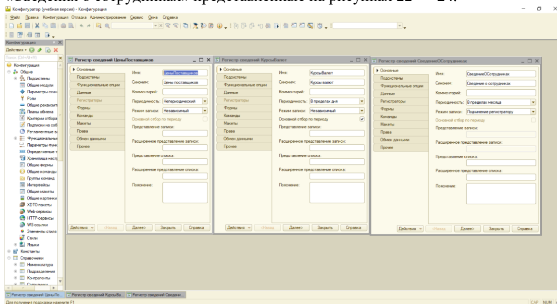
Рисунок 22 – Регистры сведений
