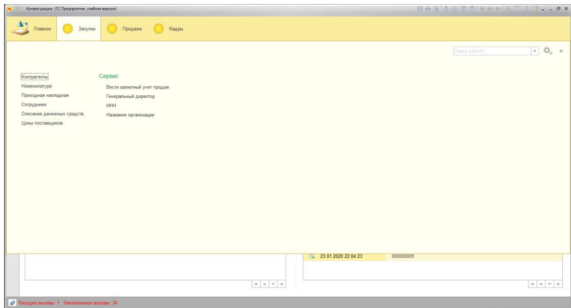
Рисунок 33 – Вкладка «Закупки»
