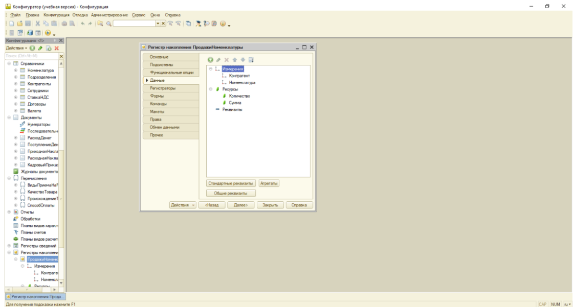
Рисунок 20 – Данные регистра
