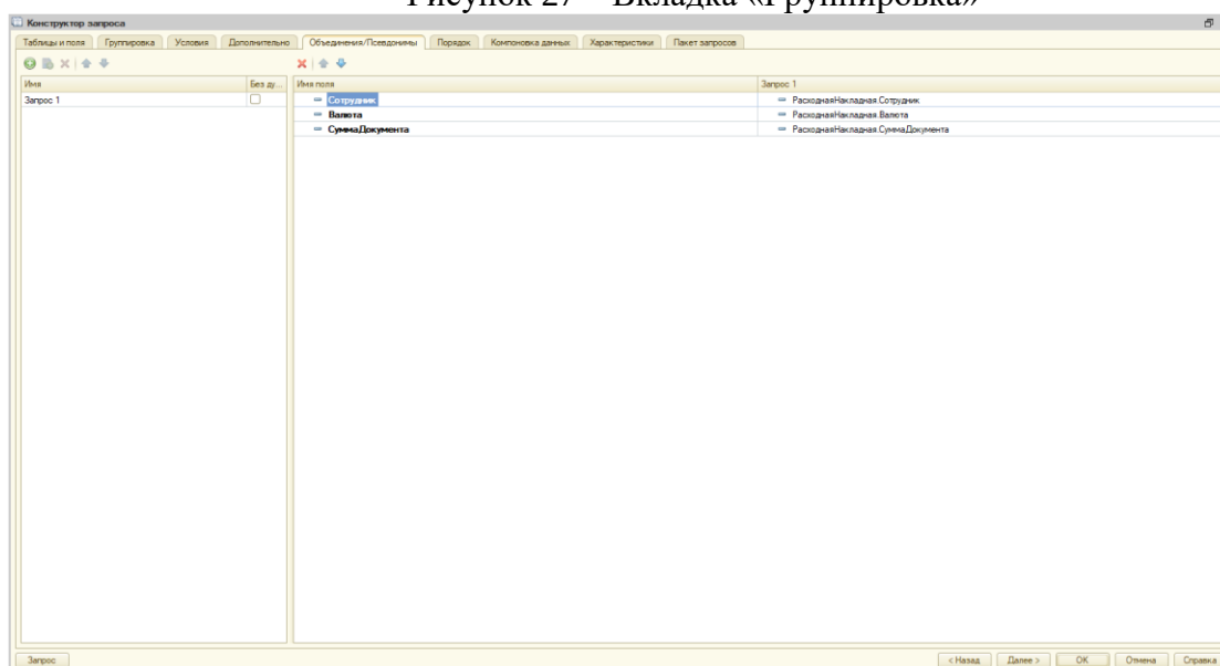
Рисунок 28 – Вкладка «Объединение/псевдонимы»
