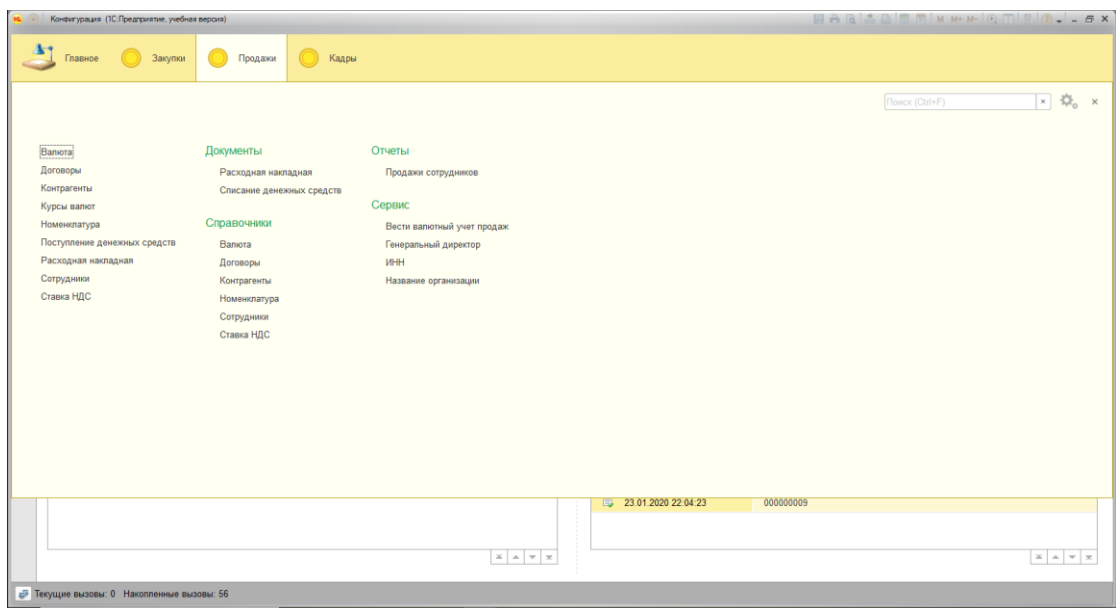
Рисунок 35 – Вкладка «Продажи»
