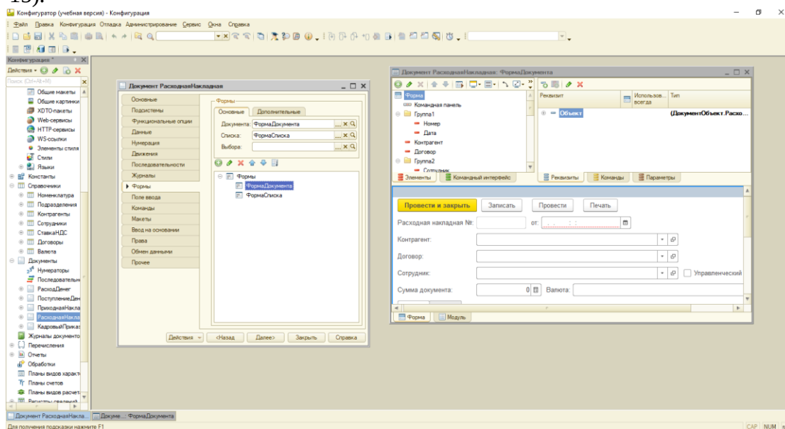
Рисунок 12 – Форма документа
