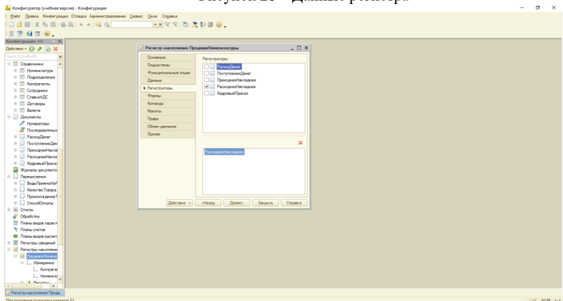
Рисунок 21 – Вкладка регистраторы
