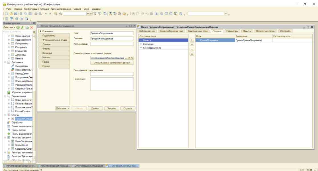
Рисунок 30 – Вкладка «Ресурсы»
