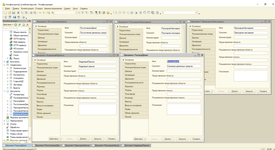
Рисунок 10 – Документы
