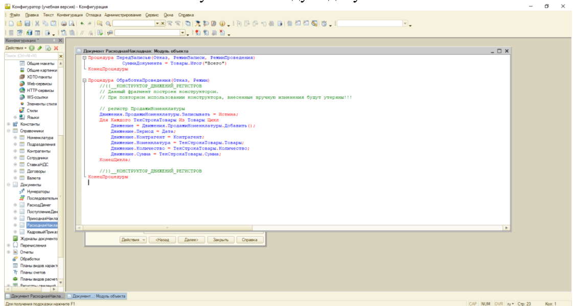
Рисунок 14 – Модуль объекта
