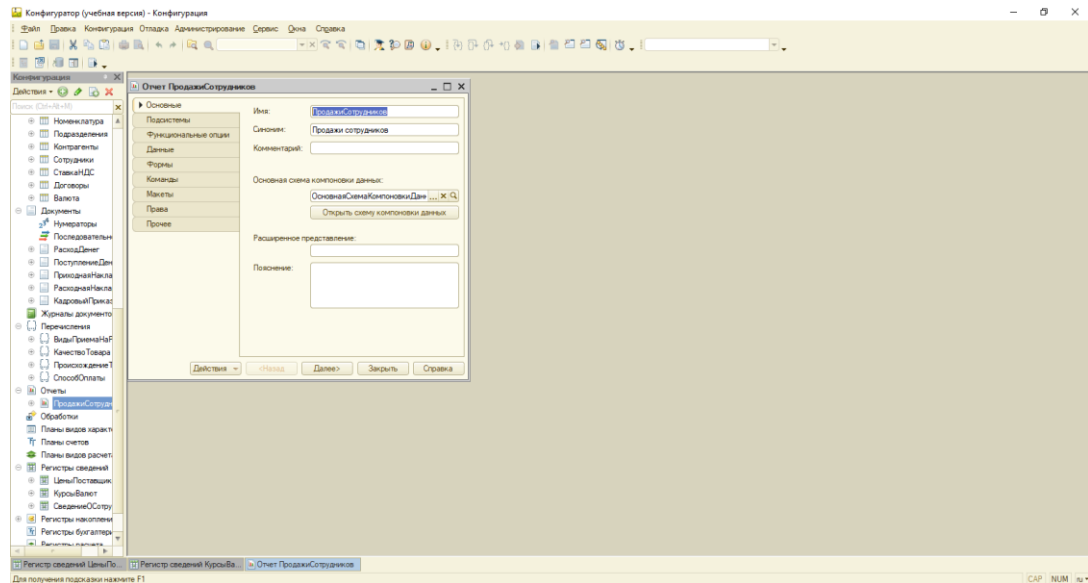
Рисунок 25 – Отчёт
