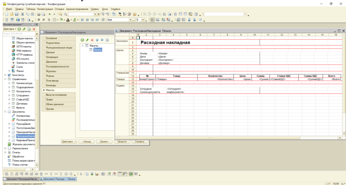
Рисунок 16 – Макет печати
