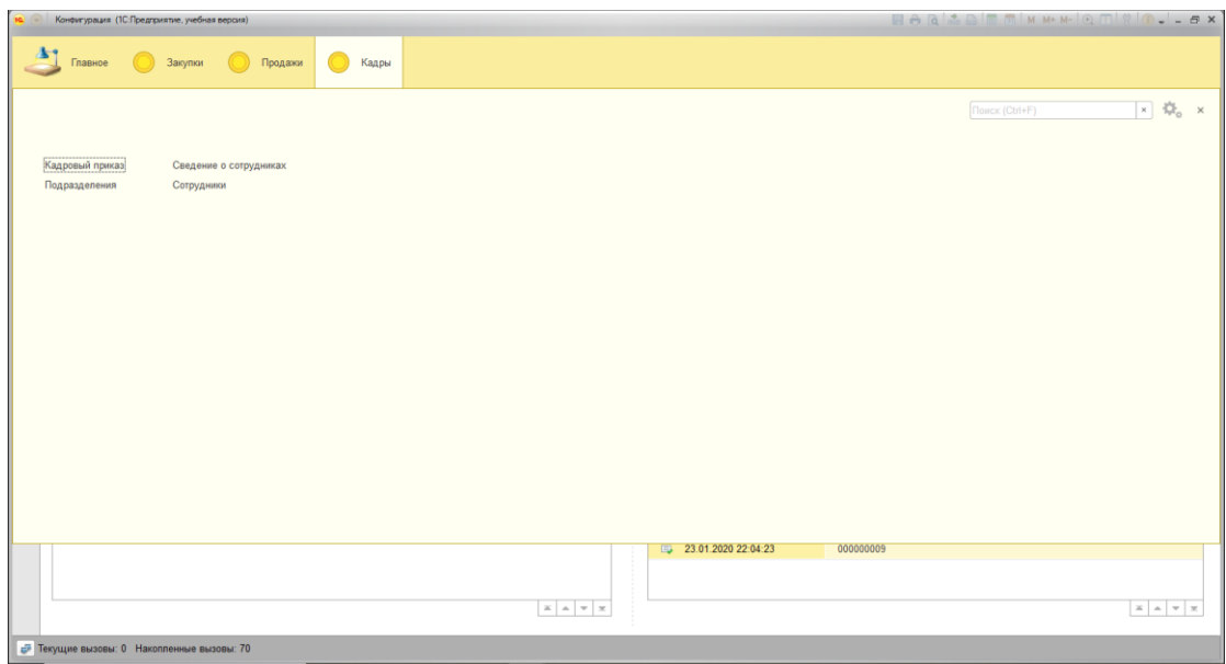
Рисунок 39 – Вкладка «Кадры»
