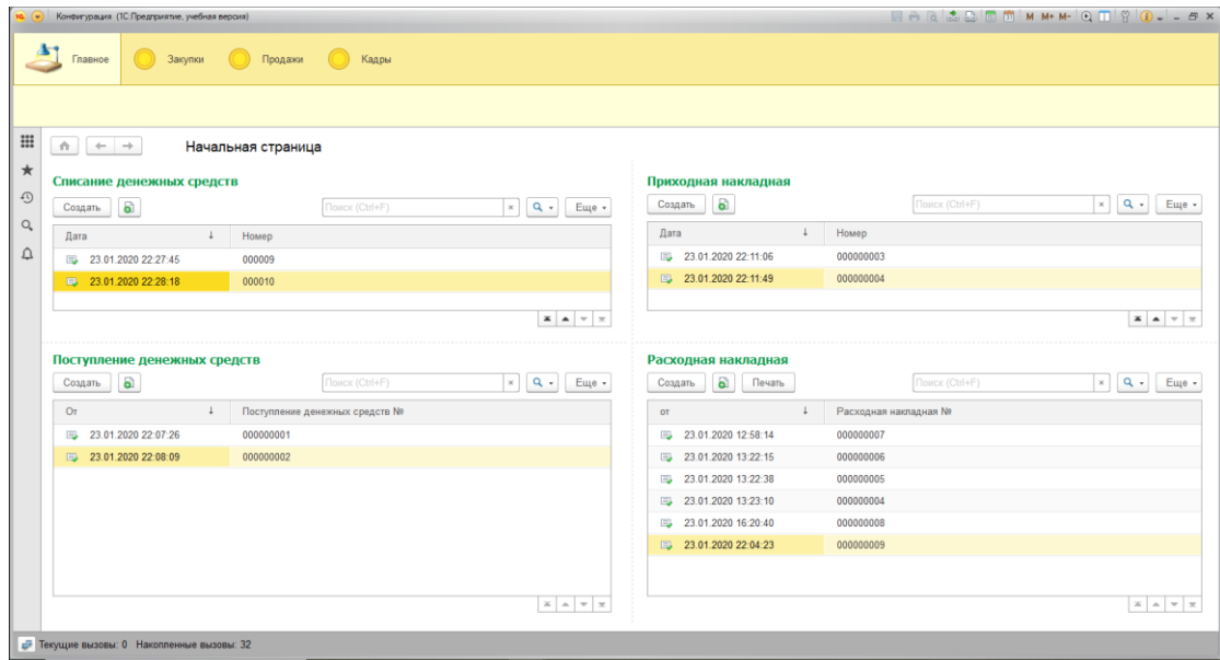
Рисунок 32 – Рабочий стол
