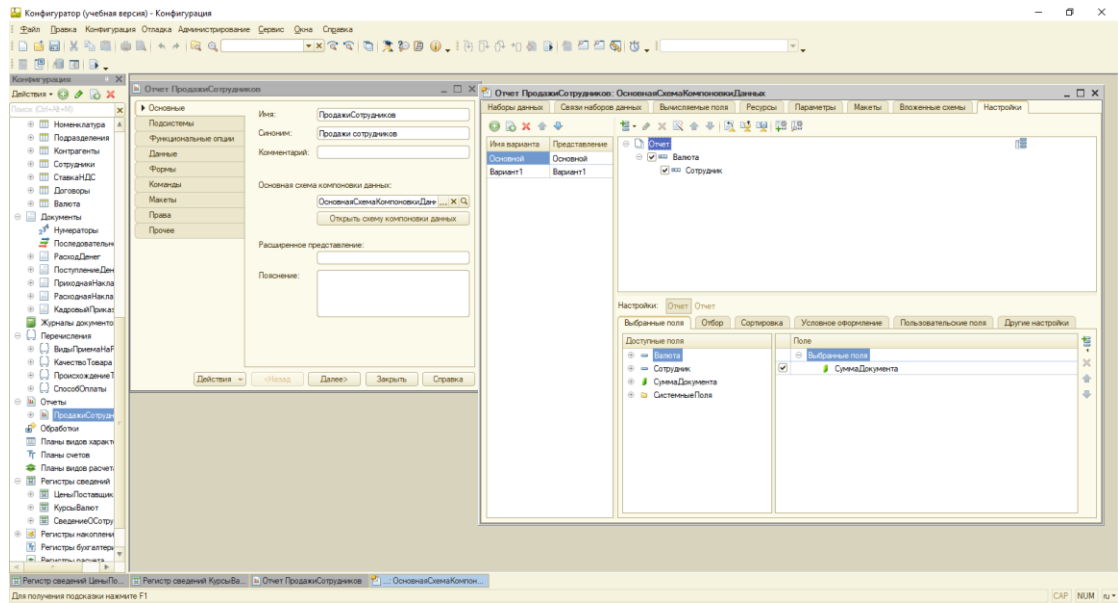
Рисунок 31 – Вкладка «Настройки»
