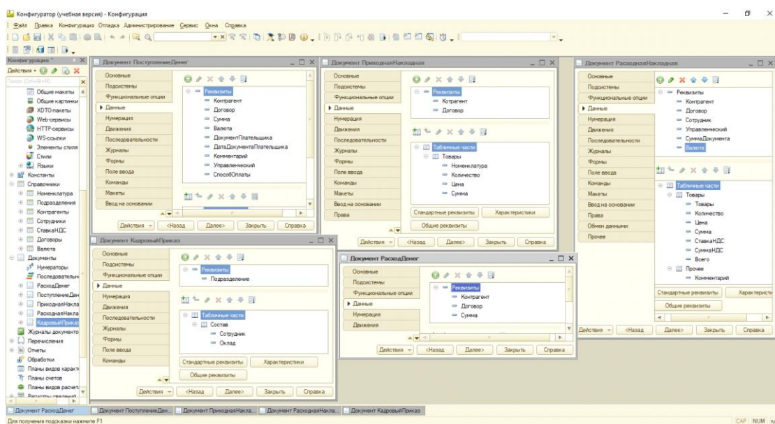
Рисунок 11 – Вкладка «Данные»
