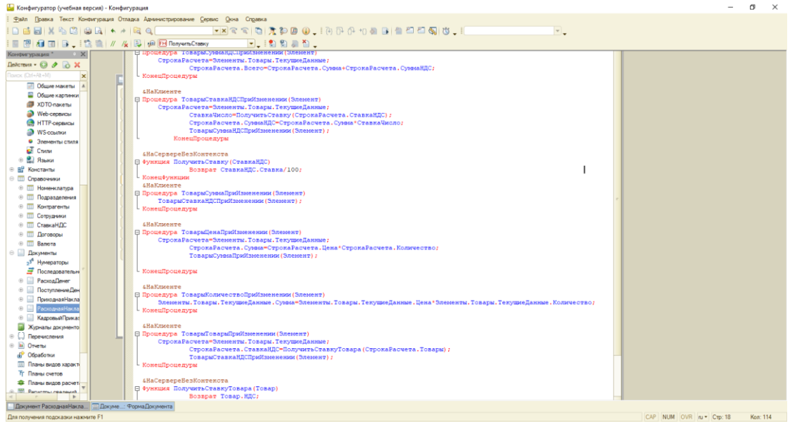
Рисунок 13 – Модуль документа
