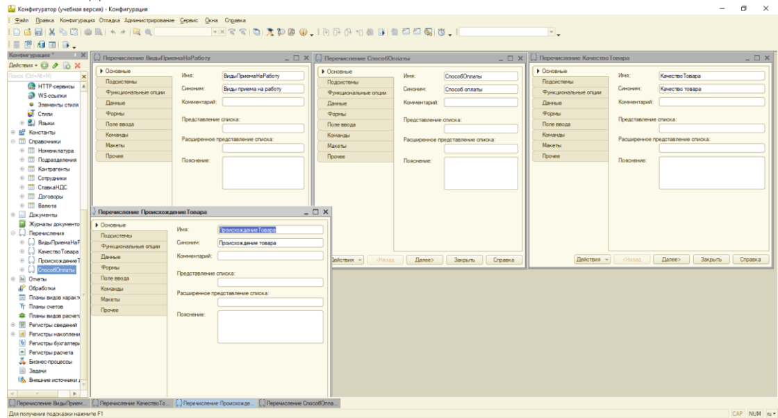
Рисунок 17 – Перечисления
