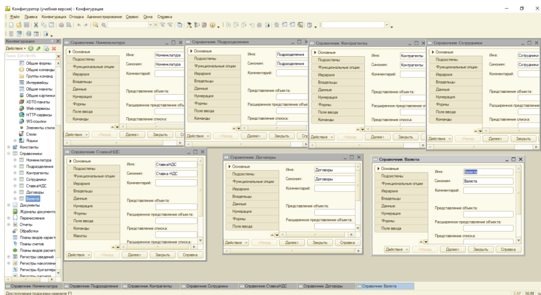
Рисунок 9 - Справочники
