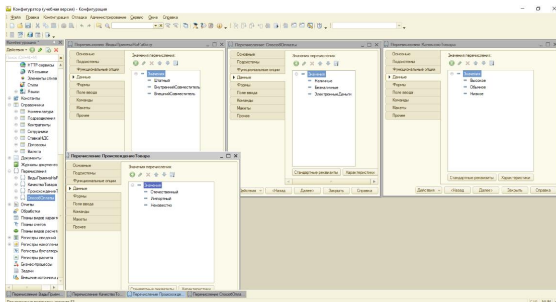
Рисунок 18 – Данные перечислений
