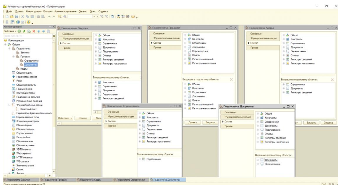
Рисунок 8 – Подсистемы
